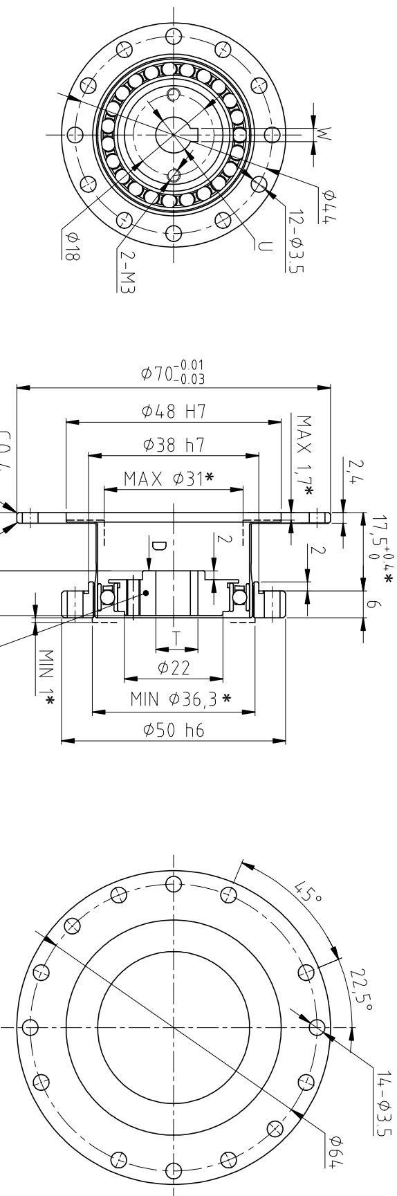
Wave generator-A
